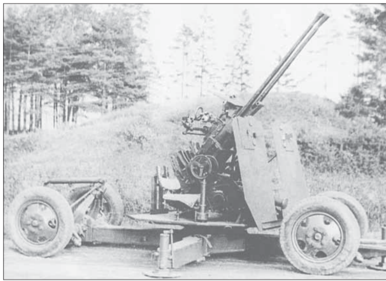
Одна из последних разработок завода — спаренная 25-мм зенитная установка 94-КМ. 1944 год.
